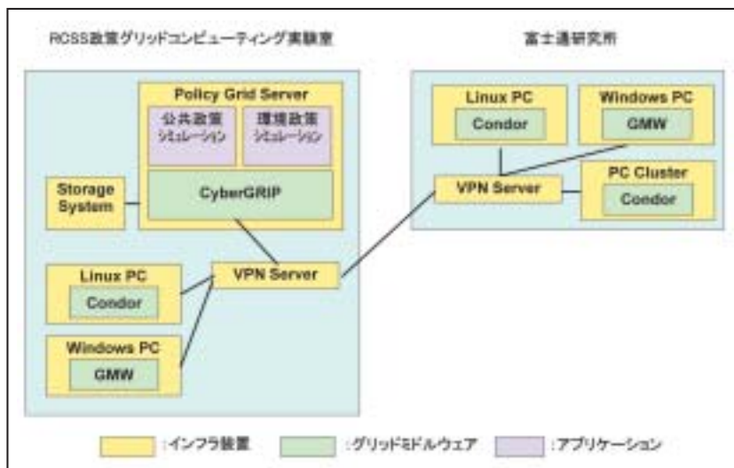
図1:商用プロバイダを介した政策グリッドシステム
