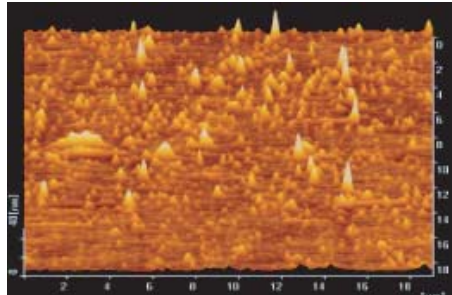
図3 フェムト秒レーザーによるナノテクスチャー
