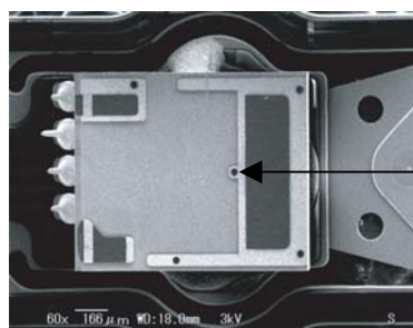
図2 ナノテクスチャー付スライダ
